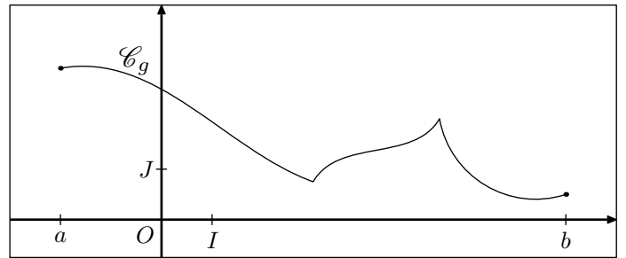
g non-dérivable sur [a; b]
