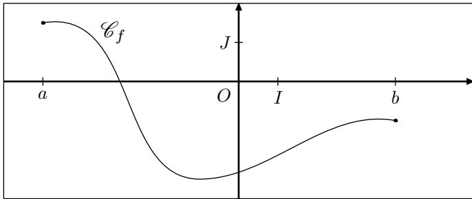
f dérivable sur [a; b]
