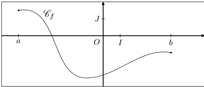
f dérivable sur [a; b]
